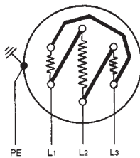
Δ Схема для 3 x 230 В (трифазний струм)
