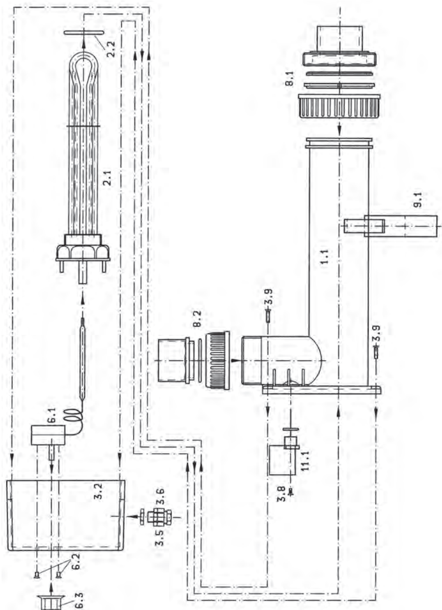
Малюнок: креслення EWT 80-81
