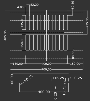
VISTA DALL'ALTO ABOVE VIEW VUE DESSUS VISTA SUPERIOR
