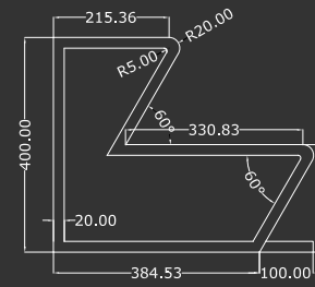
VISTA LATERALE SIDE VIEW VUE LATÉRALE
