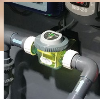
Встановлення хлоратора Installation of the chlorinator
